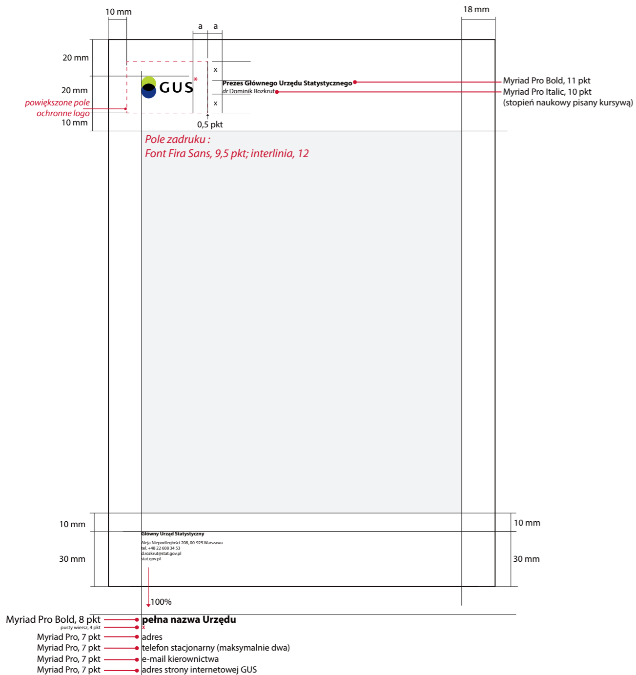
7.2.7. Schemat rozmieszczenia danych na papierze firmowym kierownictwa GUS – schemat w skali 1:2
