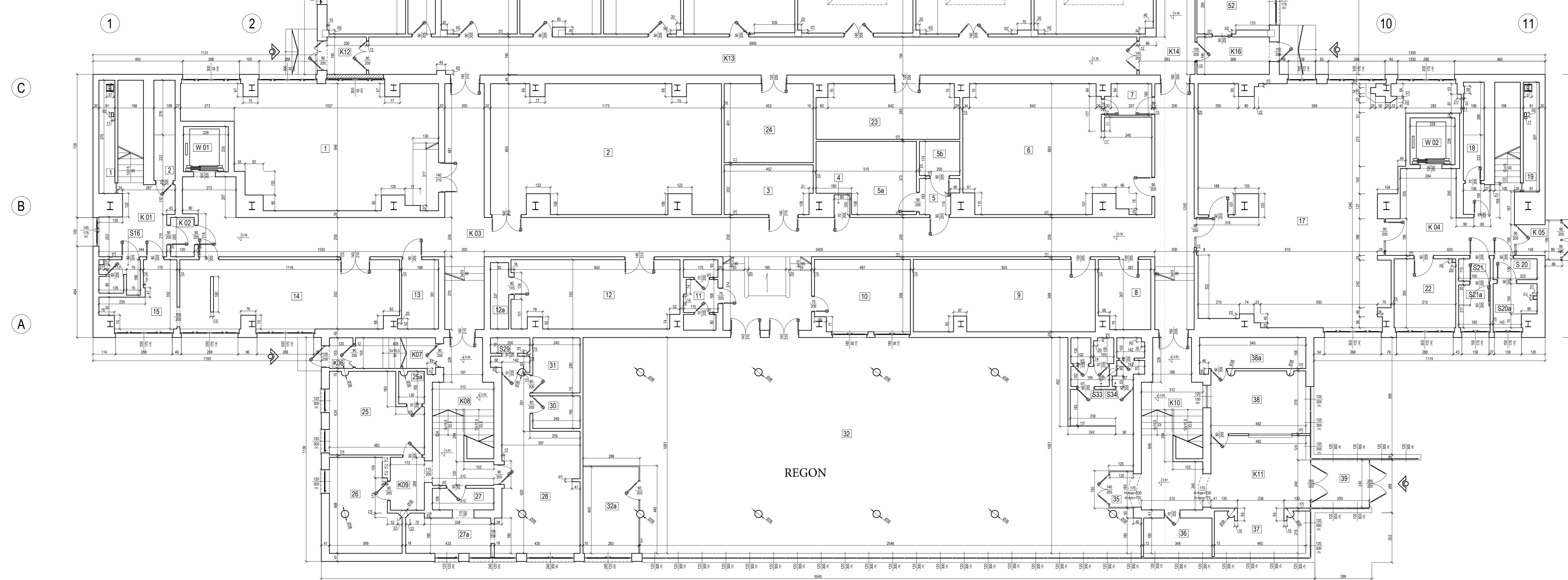
RZUT PARTERU
